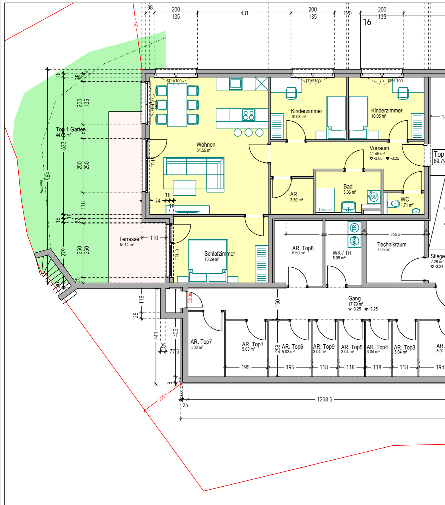
Grundriss 1:100
