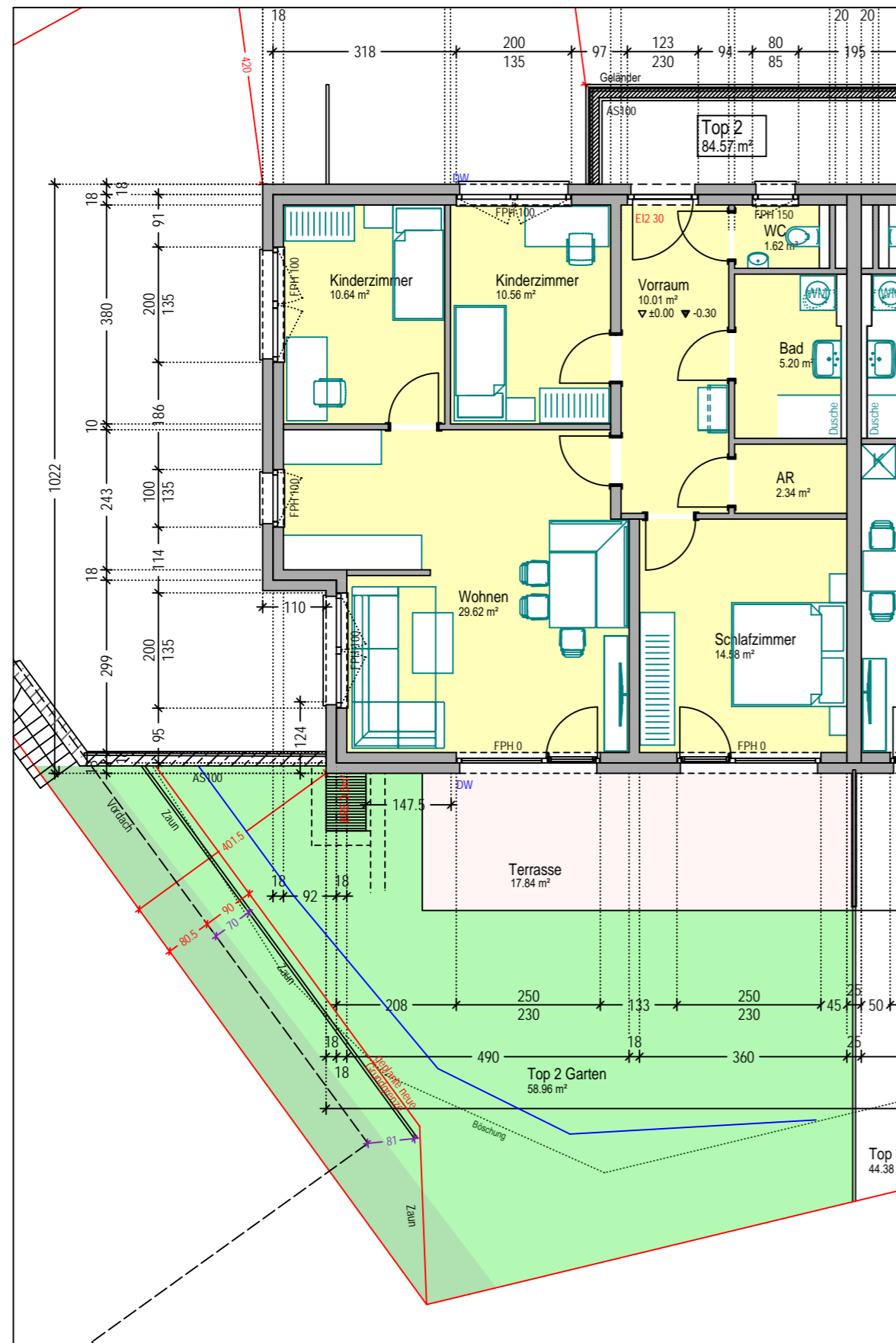
Grundriss 1:100
