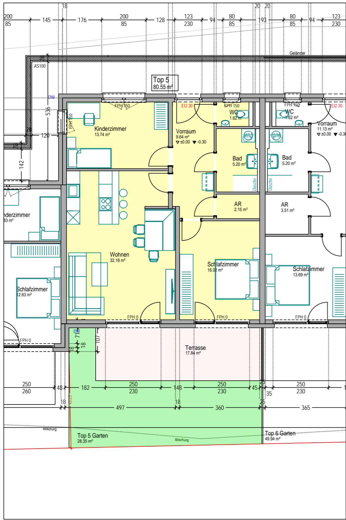
Grundriss 1:100
